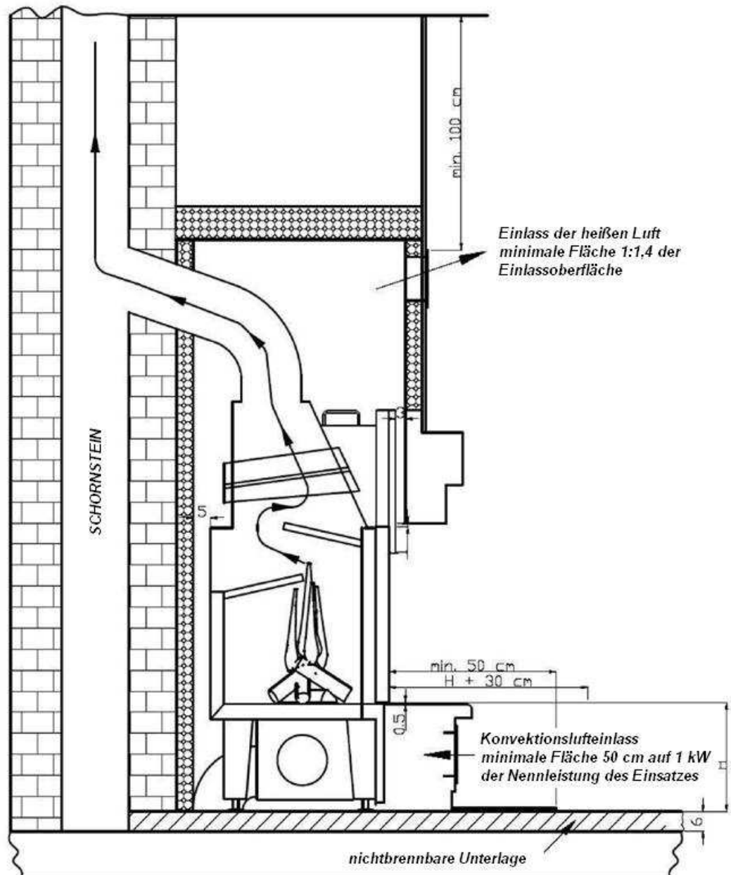
Abb. 1.3. Der Mindestraum um den Einsatz und um das Gehäuse
