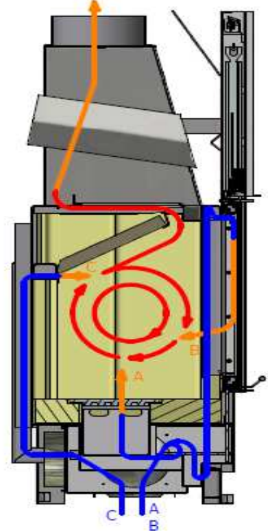
Abb. 1.7. Luftumwälzung: A-Luft unter den Rost C-Sekundärluft, B-Luftvorhang
